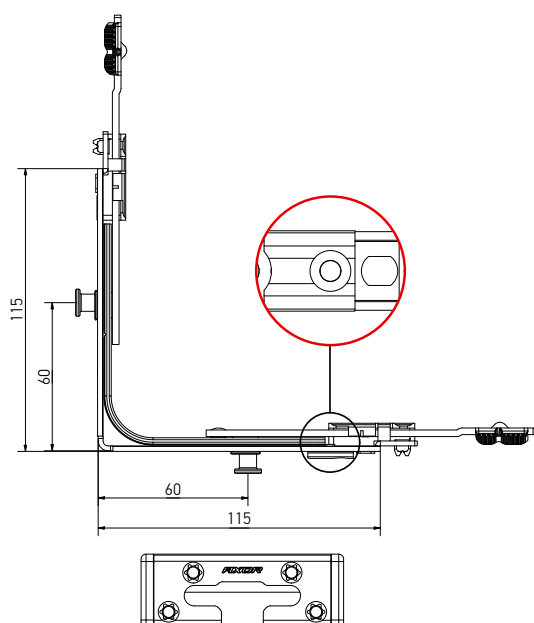
Кутова передача, нижня, 2 MR, 115×115
