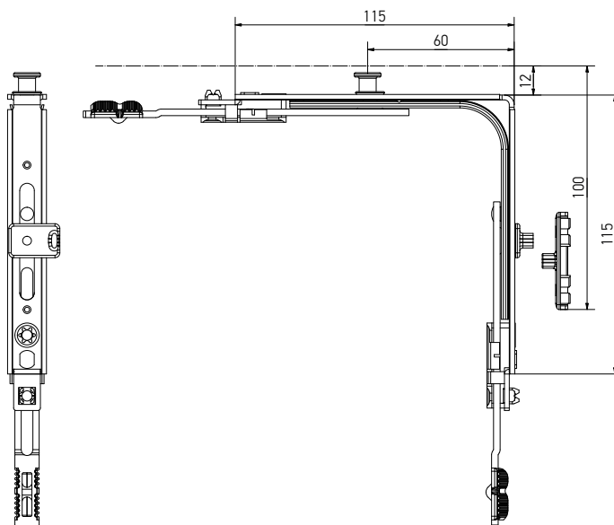
Кутова передача для ступеневого провітрювання, 1 MR, 115x115
