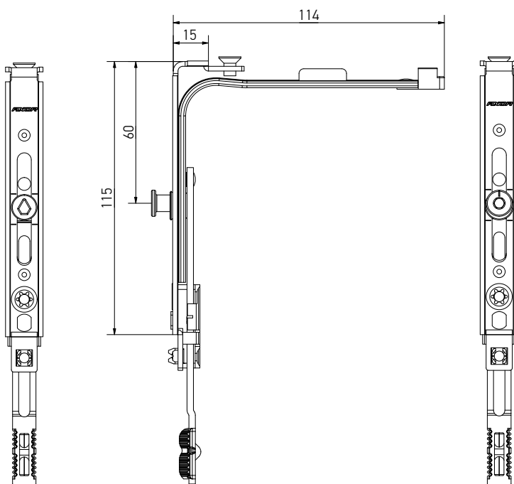
Кутова передача вузька, 1 MR, 115x15
