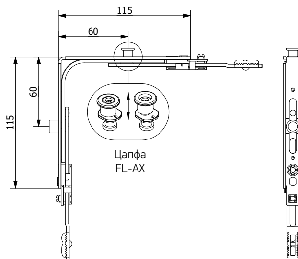
Кутова передача, нижня, 1FX +MAGNET
