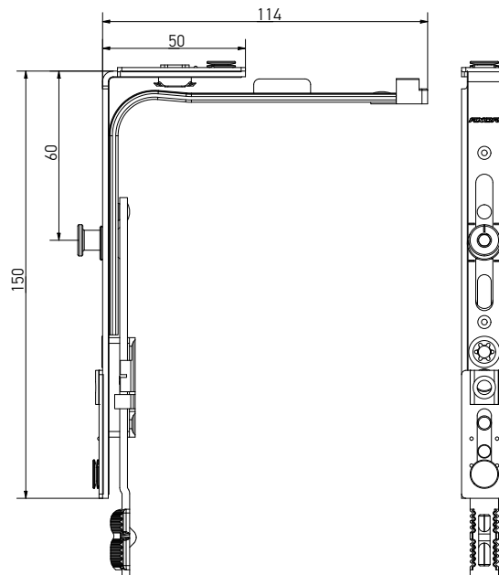
Кутова передача вузька, 1 MR, 50x150
